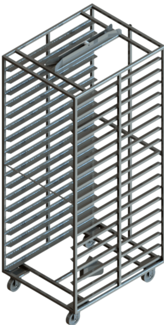
ESQUELETO PARA FORNOS ROTATIVO
